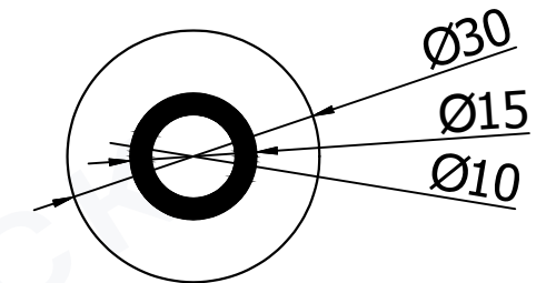
Деталь 2 (вид снизу)
