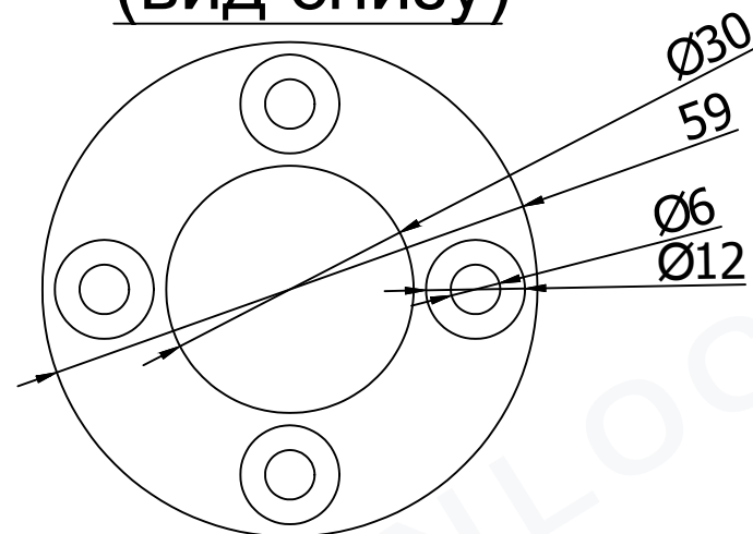
Деталь 1 (вид снизу)
