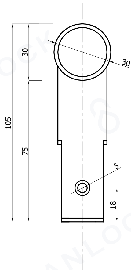
фронтальный вид
