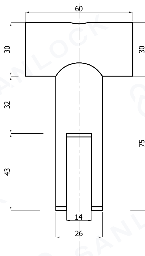
вид сбоку
